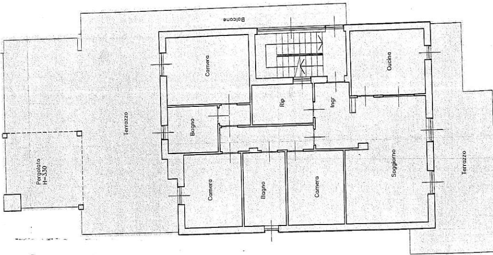
PIANTA PIANO PRIMO H=290
